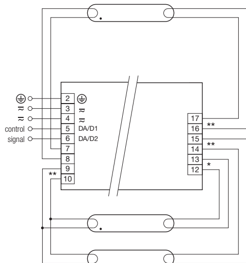
PCA T8 EXCITE Ip xitec 3x18W
